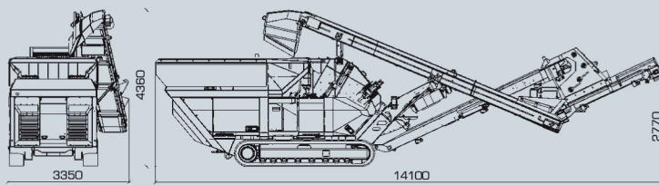
Posición de operación OS100 RFB100
