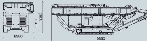
Posición de transporte OS100 RFB100
